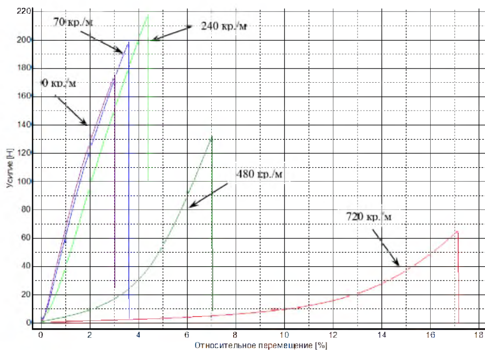
Рисунок 2 – Изменение характера диаграмм растяжения нити СВМПЭ 66 текс при различной величине крутки Figure 2 – Changing features stretching diagrams of the UHMWPE thread 66 tex at different twist values
