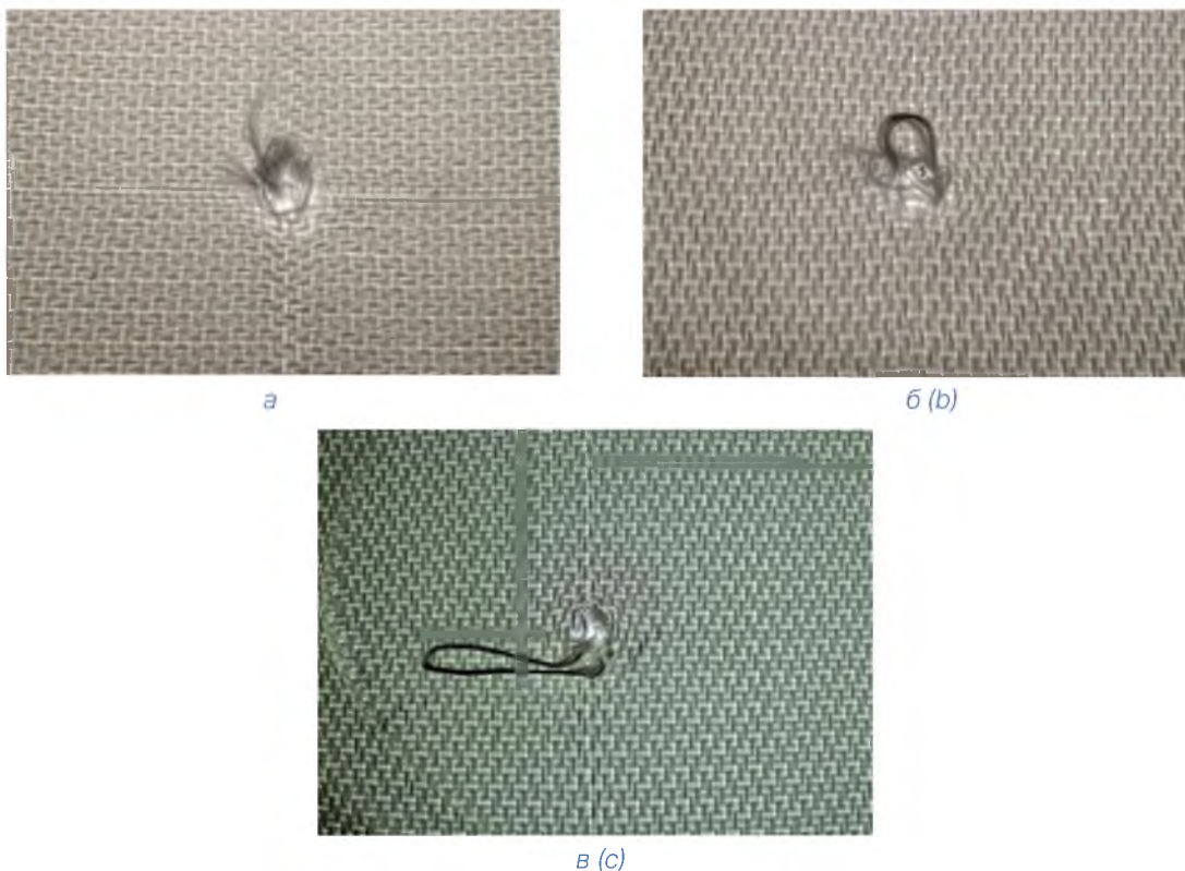
Рисунок 9 – Фотографии тканей в местах прокола: а – полиэфирная ткань с прижимным утком; б – полиэфирная ткань с комбинированным соединением слоев; в – СВМПЭ ткань с комбинированным соединением слоев
