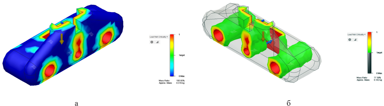
Рисунок 4 – Пример анализа детали «каретка»: а – изометрия с представлением нагруженных элементов; б – изометрия скрытой части, которая не подвергается нагрузкам
