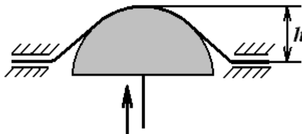
Рисунок 1 – Растяжение образцов полусферическим пуансоном
