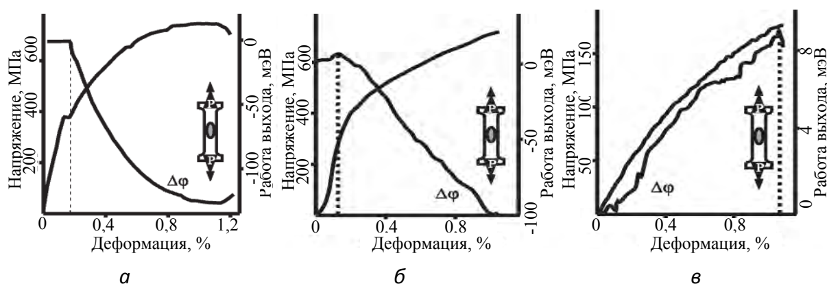
а – Ст. 45, б – А5М, в – СЧ 18-31 Рис. 1. Изменение работы выхода электрона при одноосном растяжении
