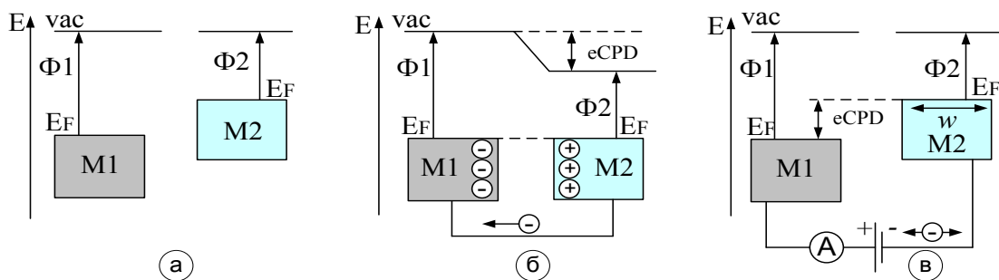
Рис. 1. Процесс измерения контактной разности потенциалов зондом Кельвина
