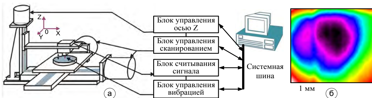
Рис. 2. Структурная схема экспериментальной установки (а), топология работы выхода электрона при точечном нагружении
