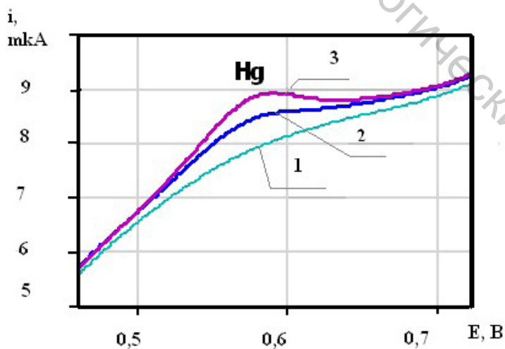
1 – фонового электролита (0,0175 моль/дм 3 H 2 SO 4 + 0,002 моль/дм 3 KCl); 2 – пробы образца жидкого туалетного мыла № 1 (Helr «Зеленый чай»); 3 – пробы образца жидкого туалетного мыла № 1 с добавкой стандартного раствора, содержащего 2 мг/дм 3 Hg
