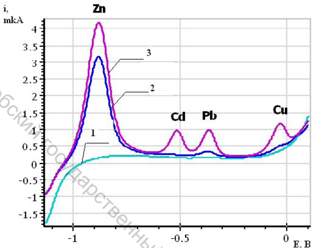
1 – фонового электролита (0,35 М водный раствор муравьиной кислоты); 2 – пробы образца жидкого туалетного мыла № 8 («Семейное»); 3 – пробы образца жидкого туалетного мыла № 8 с добавкой стандартного раствора, содержащего по 2 мг/дм 3 Cd, Pb, Cu и 3 мг/дм 3 Zn
