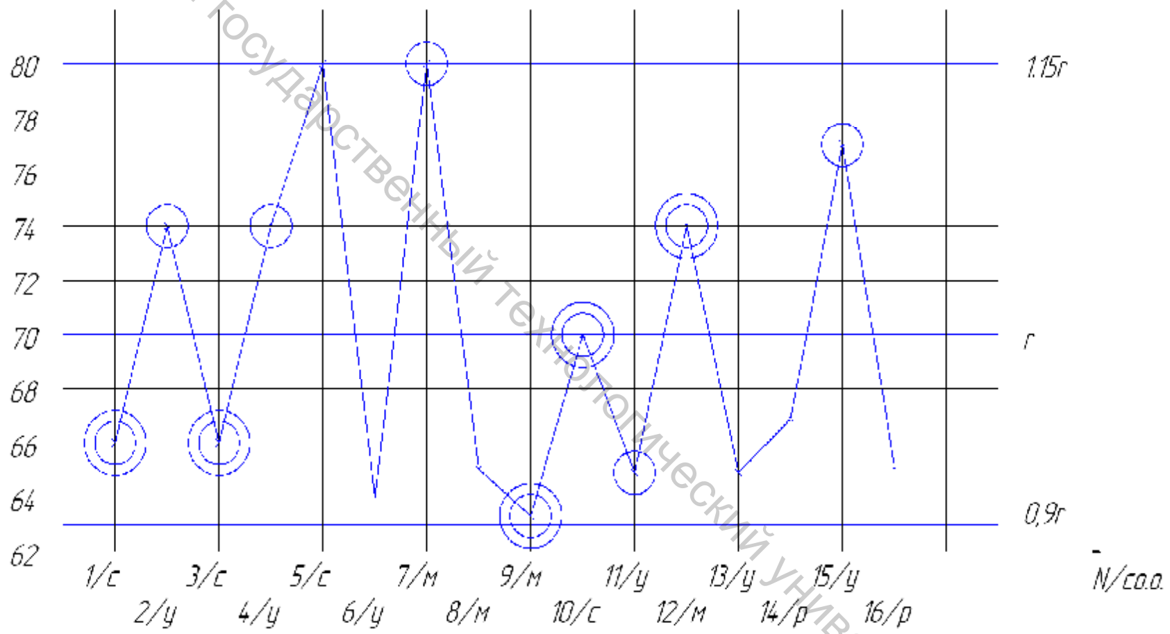
Рисунок И – График согласования
