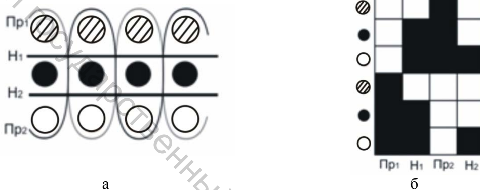
Рисунок 4 – Односторонний однолицевой пояс (эффект «броше» № 2): а) продольный разрез; б) переплетение для насечки карт
