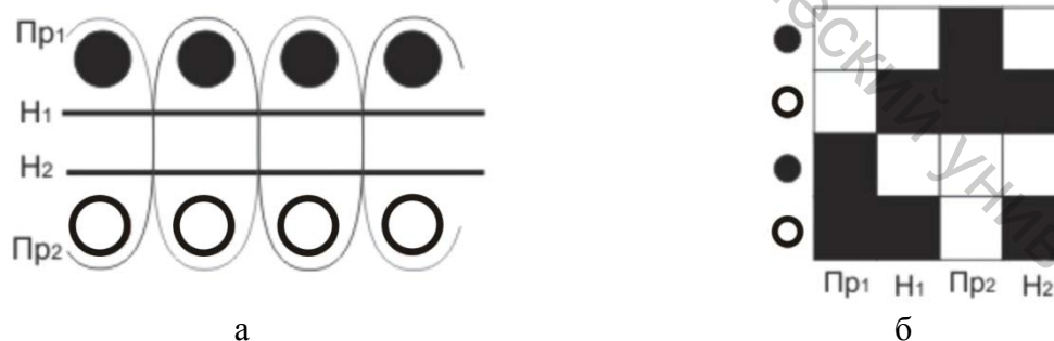
Рисунок 2 – Односторонний однолицевой пояс (цветовой эффект № 2):
