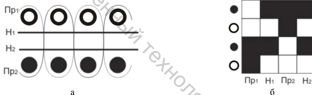
Рисунок 1 – Односторонний однолицевой пояс (цветовой эффект № 1):
