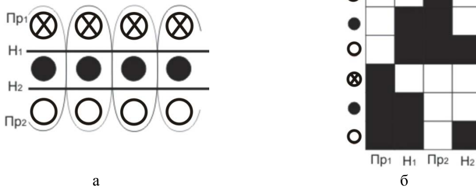
Рисунок 3 – Односторонний однолицевой пояс (эффект «броше» № 1): а) продольный разрез; б) переплетение для насечки карт
