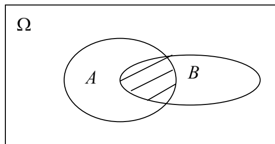
Рисунок 2.1.2 – Пересечение
