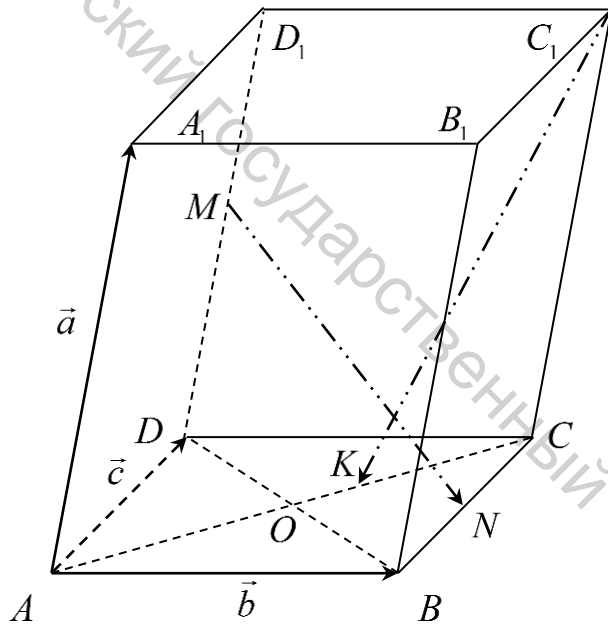
Рисунок 3.2.3 – Параллелепипед
