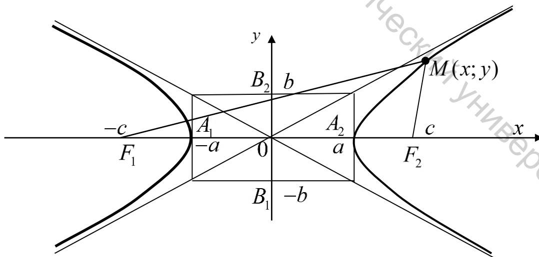
Рисунок 12.1.3 – Гипербола
