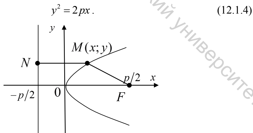
Рисунок 12.1.4 – Парабола
