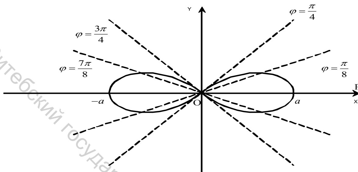
Рисунок 12.2.1 – Двухлепестковая роза
