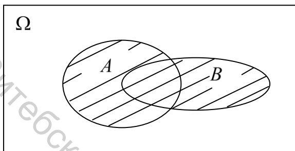
Рисунок 2.1.1 – Объединение
