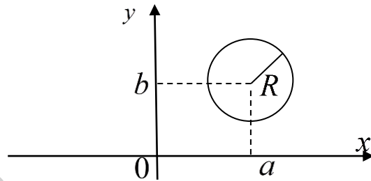
Рисунок 12.1.1 – Окружность
