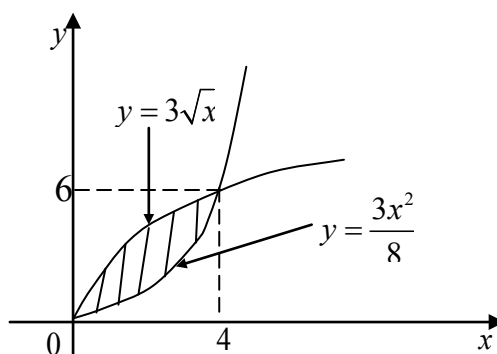
Рисунок 3.6 – Область интегрирования D для примера 2
