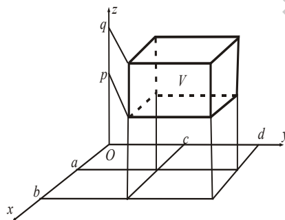
Рисунок 3.13 – Случай прямоугольной области
