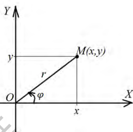
Рисунок 1.1 – Изображение комплексного числа на плоскости
