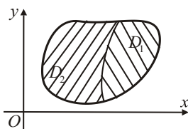
Рисунок 3.2 – Область D=D_1 \cup D_2
