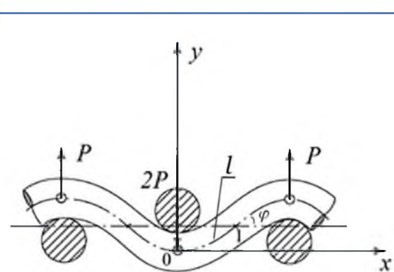
Рисунок 1 – Изгиб консольной упругой нити в структурном элементе ткани на участке 01
