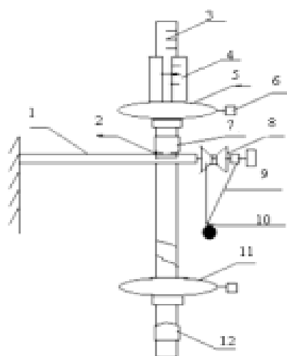
Рисунок 6.2 – Прибор ФП1А для определения ускорения свободного падения
