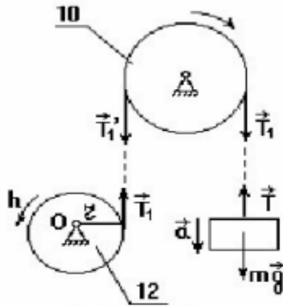
Рисунок 2.4 – Схема опыта для измерения углового ускорения маятника Обербека
