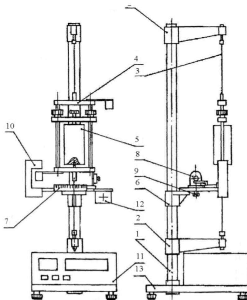
Рисунок 9.3 – Схема установки подвеса для определения момента инерции тел методом крутильных колебаний
