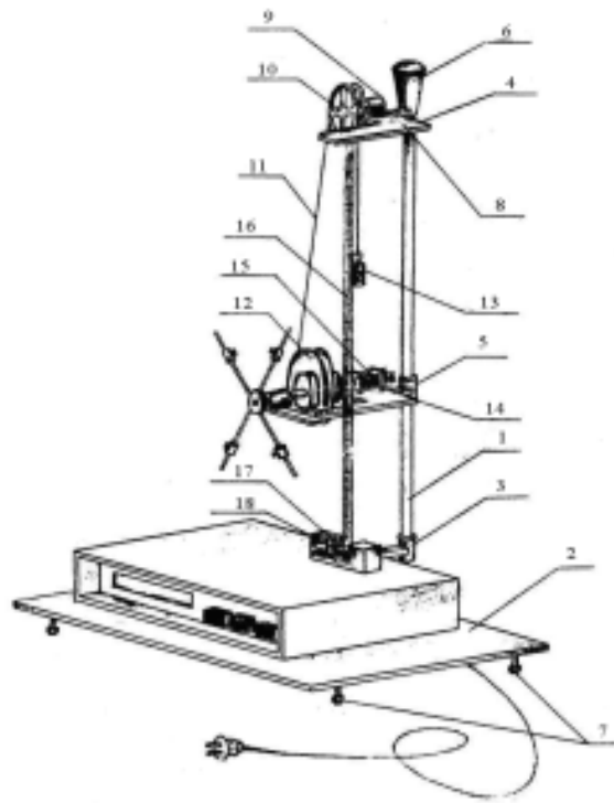
Рисунок 2.3 – Маятник Обербека
