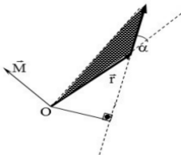
Рисунок 2.1 – Направление вектора момента силы M (правило правого винта)
