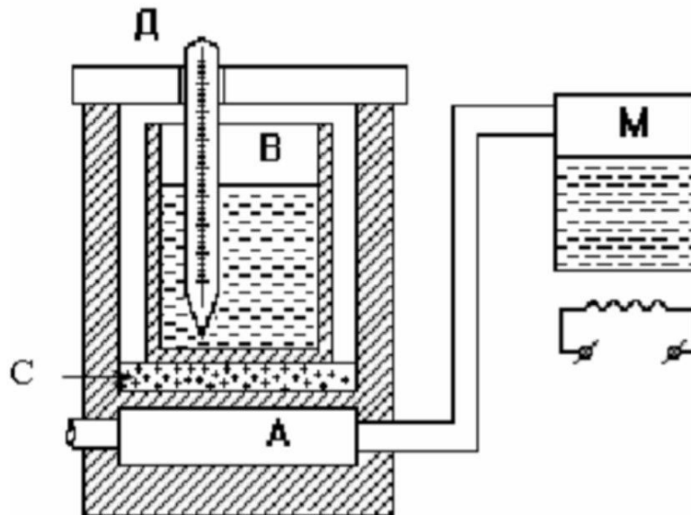
Рисунок 11.2 – Схема установки для определения коэффициента теплопроводности тел
