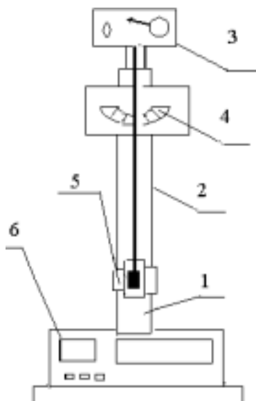
Рисунок 7.2 – Установка для изучения параметрического резонанса
