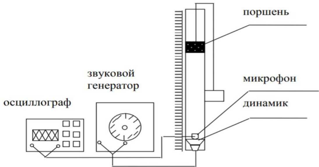
Рисунок 8.2 – Схема установки для определения скорости звука в воздухе
