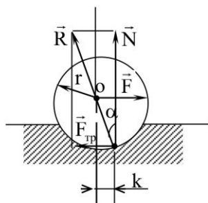
Рисунок 4.1 – Силы, действующие на цилиндр при качении
