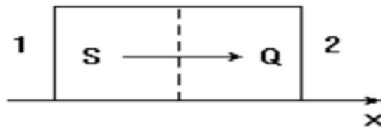
Рисунок 11.1 – Перенос теплоты Q через площадь сечением S от основания 1 к основанию 2 вдоль оси X
