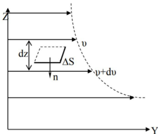
Рисунок 10.1 – Ламинарный поток в жидкости в YZ координатах
