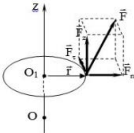
Рисунок 2.2 – Разложение силы F на три взаимно перпендикулярные составляющие
