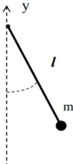
Рисунок 7.1 – Математический маятник
