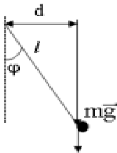
Рисунок 5.1 – Математический маятник
