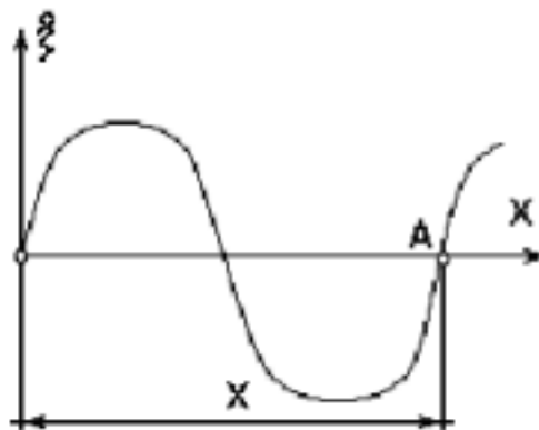
Рисунок 8.1 – Зависимость величины отклонения \zeta от положения равновесия всех частиц среды, расположенных на различных расстояниях X от источника волны
