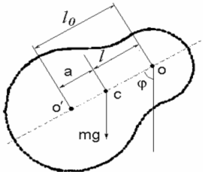
Рисунок 6.1 – Физический маятник
