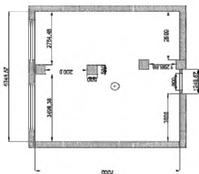
Рис. 1. Исходный план и план с возведенными перегородками
