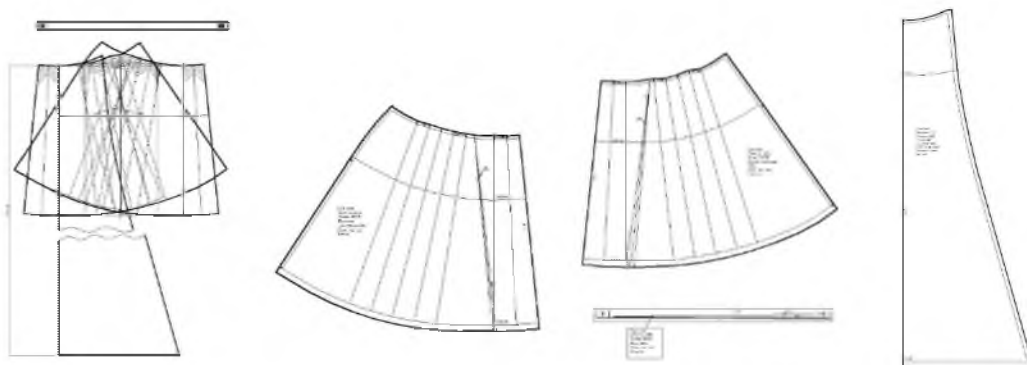
Рисунок 3. Чертеж конструкции и схемы построения чертежей лекал основных деталей модели женской юбки
