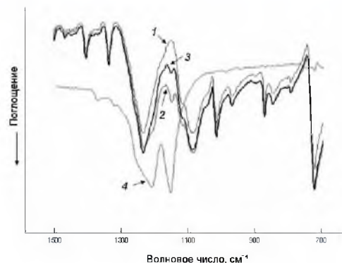
Рисунок 1 – ИК спектры (МНПВО):
