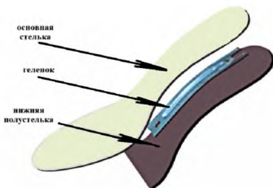
Рисунок 2 – Составные части трехслойного гибкого стелечного узла Figure 2 – Components of a three-layer flexible insole unit
