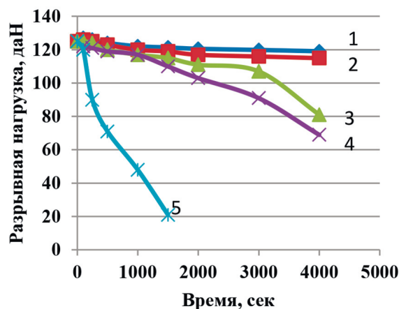
Рисунок 1 – Изменение разрывной нагрузки ткани арт. 31370ЗТ от продолжительности воздействия теплового потока плотности, кВт/м 2 : 1 – 12; 2 – 28; 3 – 37; 4 – 45 и 5 – 75 (коэффициент вариации ~ 4,0%)
