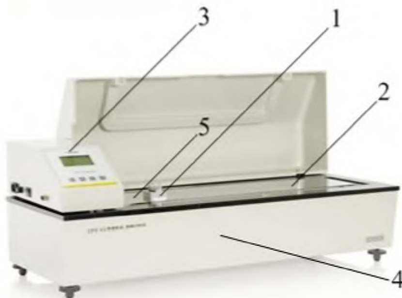
Рисунок 2 – Прибор FPT-F1
