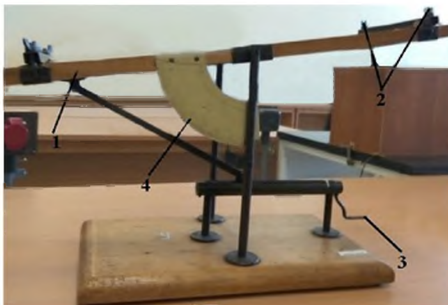
Рисунок 10 – Прибор для определения коэффициента тангенциального сопротивления методом наклонной плоскости УО «ВГУ»: 1 – подвижная платформа; 2 – винтовые зажимы; 3 – рукоятка; 4 – линейка
