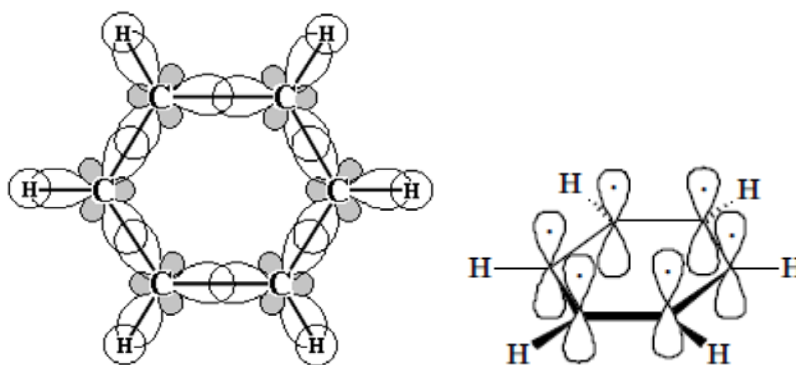
Рисунок 4.5 – Строение молекулы бензола
