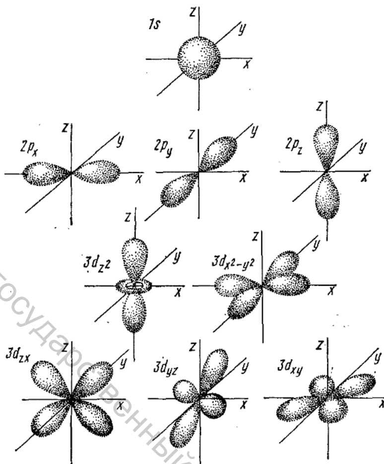
Рисунок 1.2 – Форма электронных орбиталей
