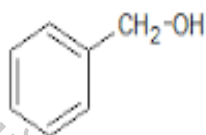
бензиловый спирт
