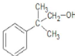
2-метил-2-фенилпропанол-1
