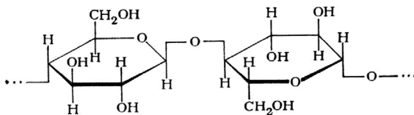
Рисунок 4.8 – Структурное звено целлюлозы
