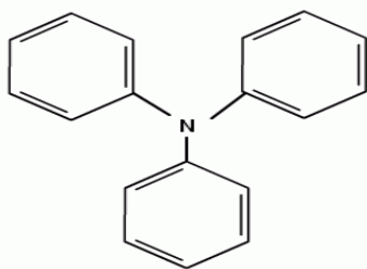
←трифениламин (третичный амин)
