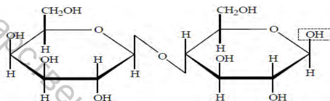
β-лактоза β-D-галактопиранозил-1,4-β-D-глюкопираноза
