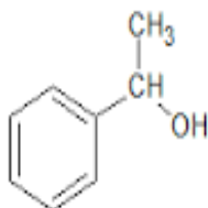
1-фенилэтанол-1
