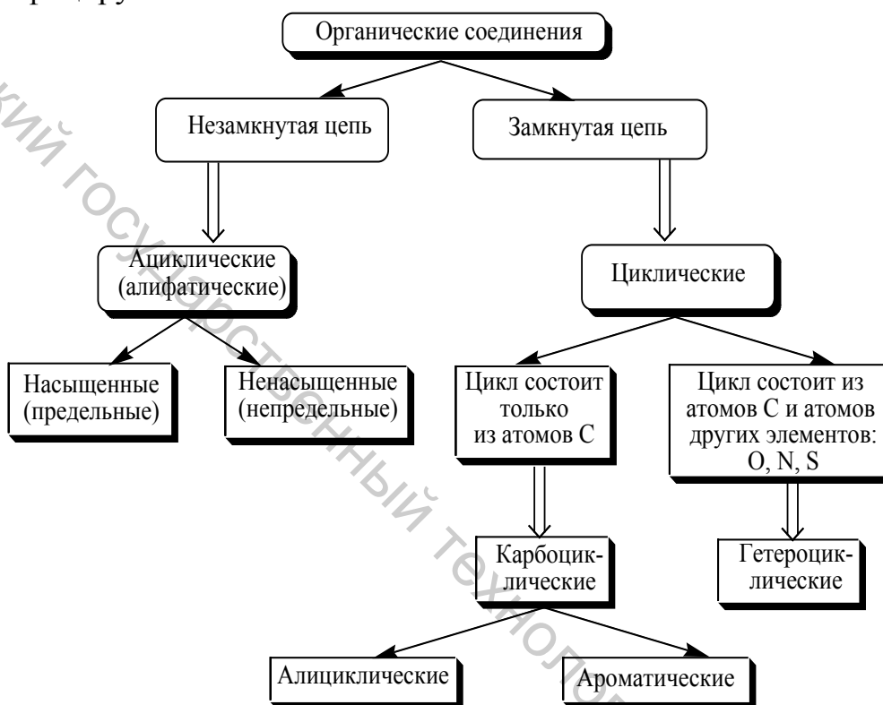
Рисунок 4.1 – Классификация органических соединений
