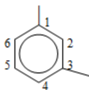
m-фенилен
