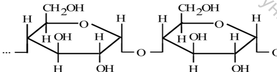
Рисунок 4.7 – Структурное звено крахмала
