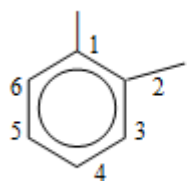
o-фенилен
