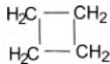
циклобутан
