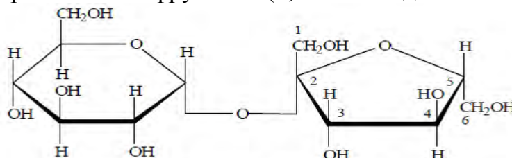
α-D-глюкопиранозил-1,2-β-D-фруктофуранозид
