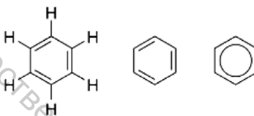
Рисунок 4.6 – Бензол
