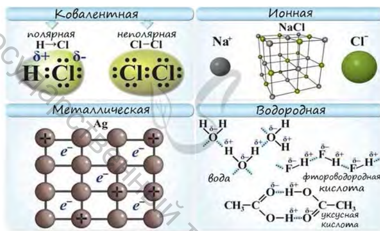
Рисунок 1.3 – Типы химических связей
