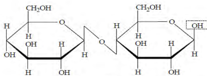
β-целлобиоза β-D-глюкопиранозил-1,4-β-D-глюкопираноза
