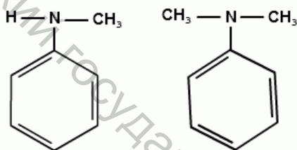
N-метиланилин
