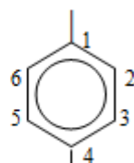
p-фенилен
