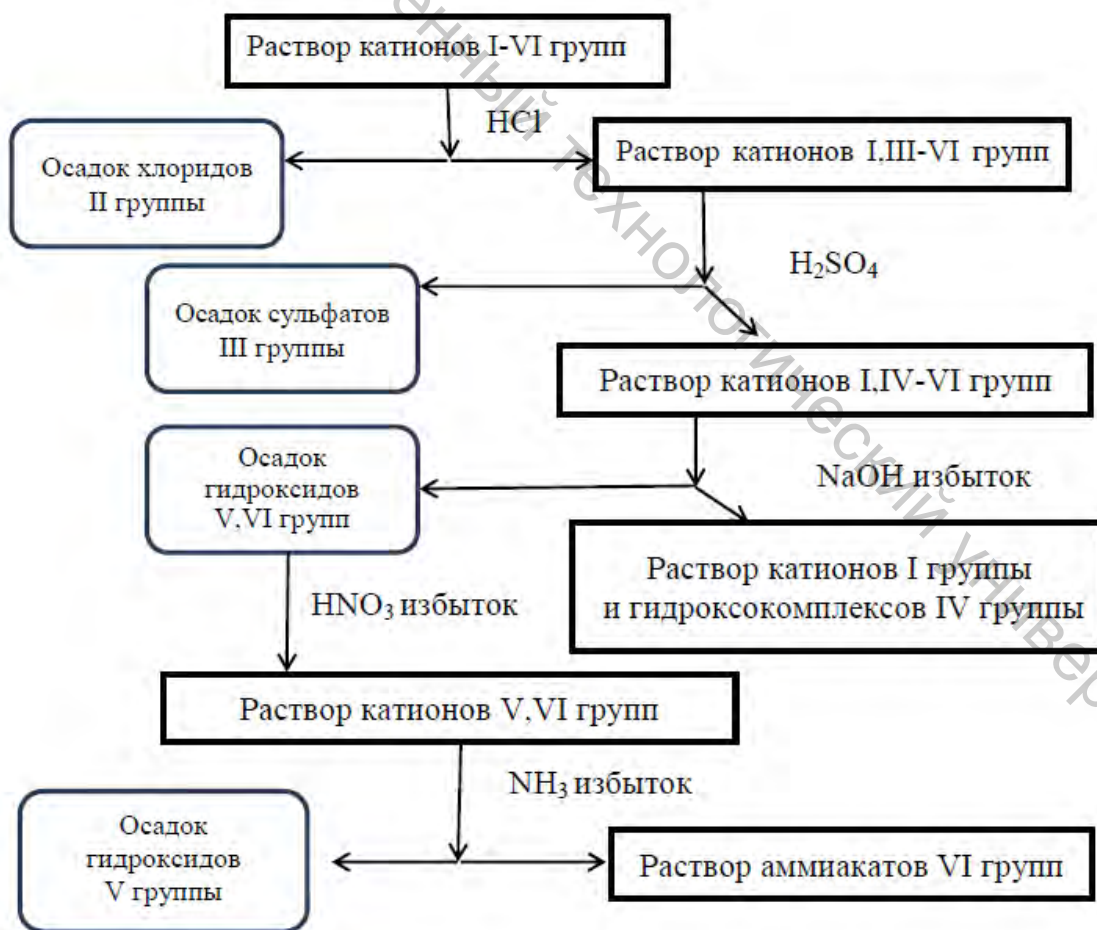
Рисунок 3.1 – Кислотно-щелочная схема анализа смеси катионов
