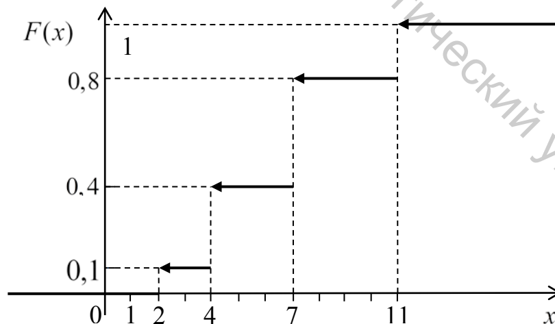
Рисунок 1 – График функции распределения
