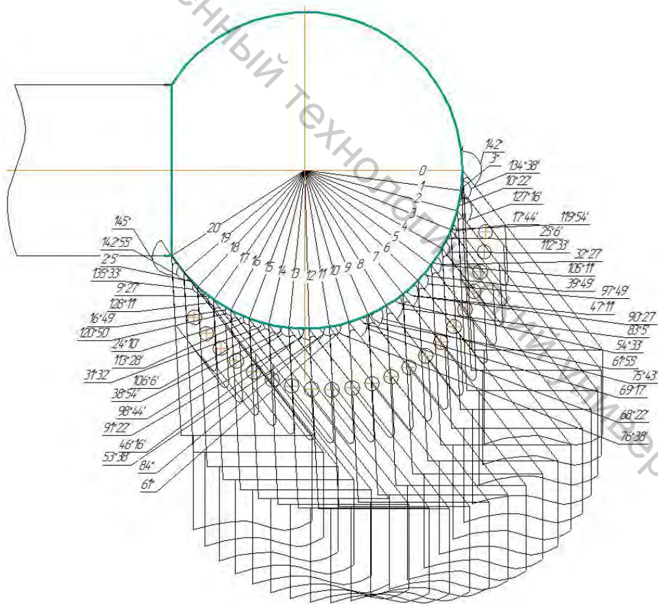
Рисунок 10 – Схема изменения главного и вспомогательного углов в плане реза
