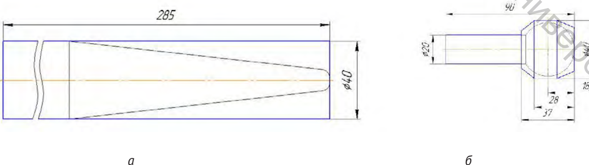
Рисунок 2 – Заготовки деталей: а) «Штырь», б) «Палец шаровой»
