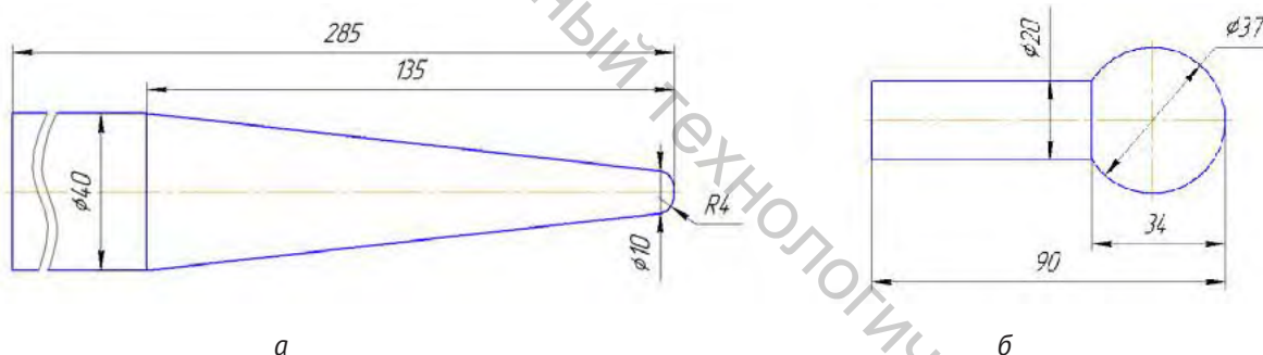
Рисунок 1 – Детали: а) «Штырь», б) «Палец шаровой»
