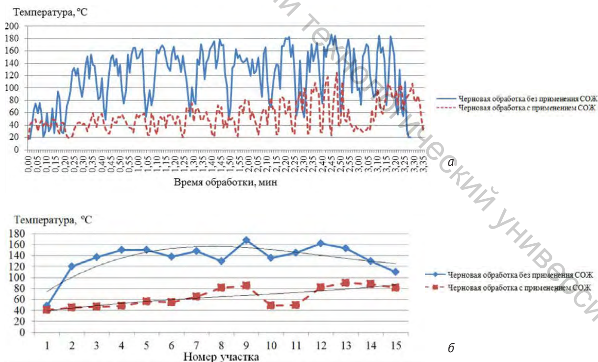
Рисунок 5 – Зависимости температуры от времени обработки (а) и на различных участках обрабатываемой конической поверхности детали (б)
