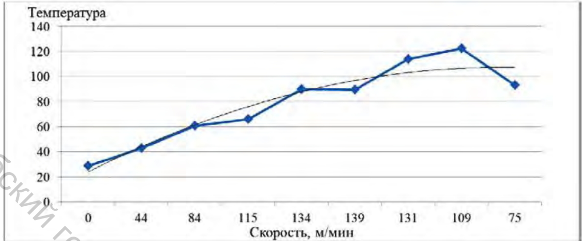
Рисунок 9 – Зависимость значений температуры от линейной скорости резания при чистовой обработке сферической поверхности с частотой вращения заготовки n = 1200 \text{ мин}^{-1} и подаче инструмента s = 0,2 \text{ мм/об}
