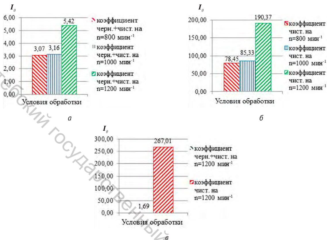
Рисунок 14 – Диаграммы приведенной интенсивности изменения температуры при различных условиях обработки сферической поверхности детали: а – черновая обработка при t = 0,8 мм; б – чистовая обработка при t = 0,8 мм; в – черновая и чистовая обработка при t = 0,2 мм
