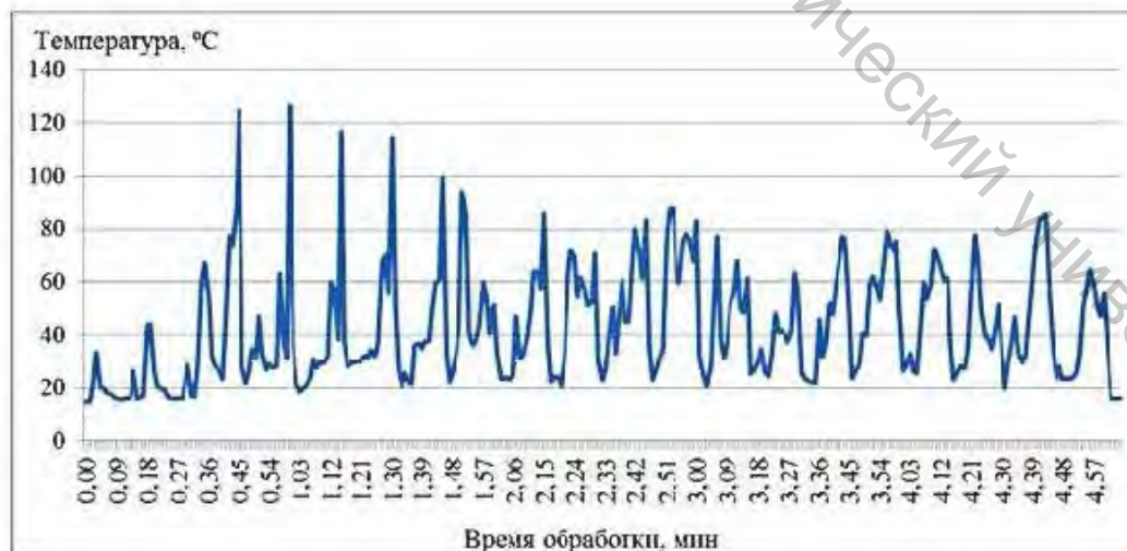
Рисунок 11 – Зависимость значений температуры от времени при черновой и чистовой обработке сферической поверхности детали
