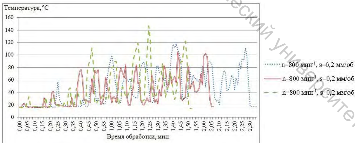
Рисунок 7 – Зависимости значений температуры от времени при обработке сферической поверхности детали
