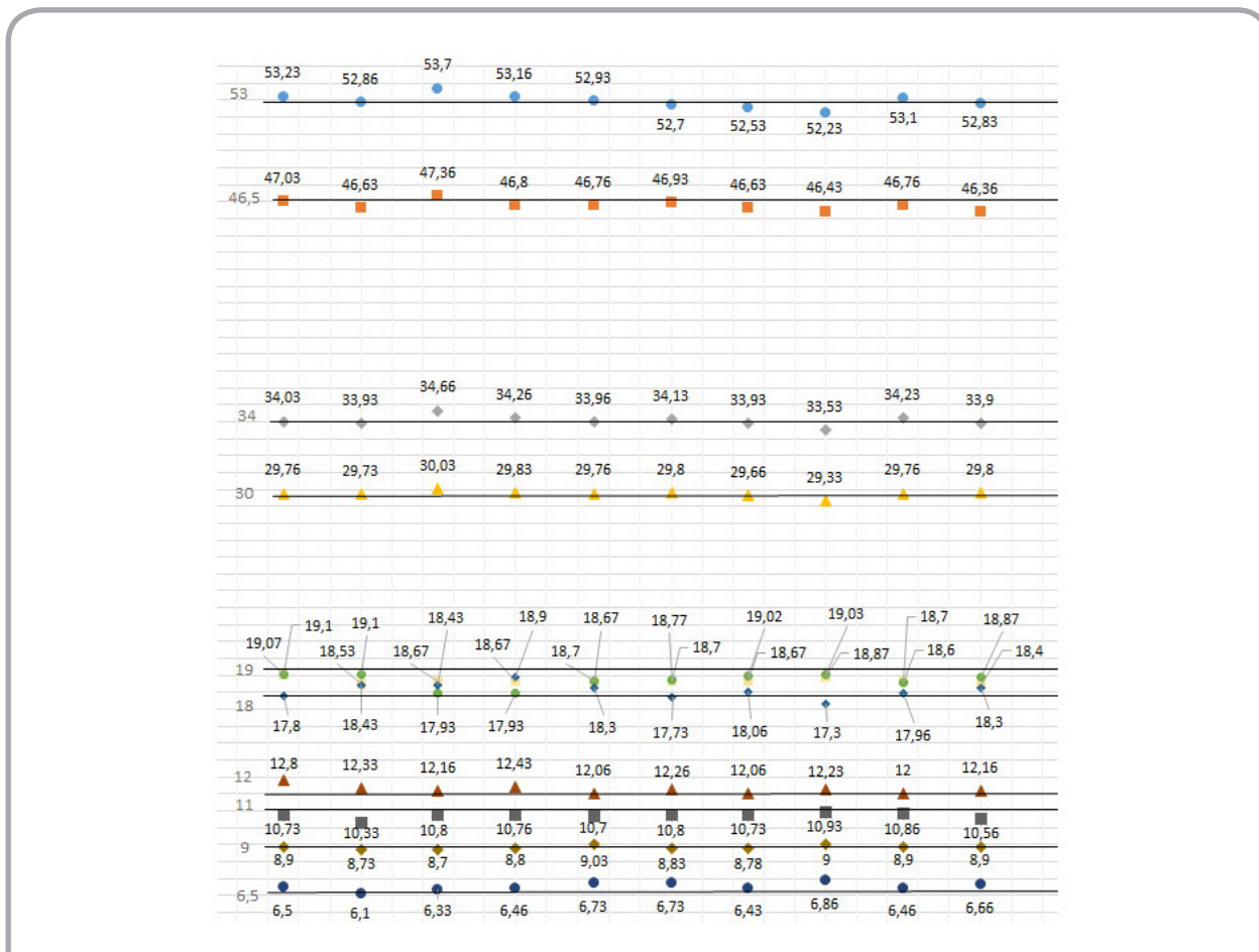
Рисунок 7 – График отклонений линейных размеров изделия от номинальных значений (сплошная линия) для различных пластиковых материалов
