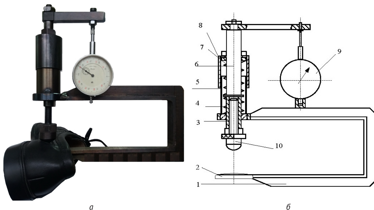
1 – скоба, 2 – кольцо, 3 – измерительный шток, 4 – фиксирующая пружина, 5 – корпуса, 6 – грузовой шток, 7 – пружина, 8 – нажимной винт, 9 – индикатор часового типа, 10 – съемный сферический наконечник
