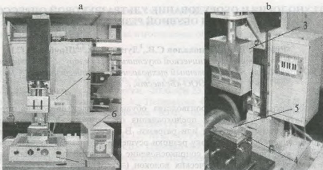
Рисунок 1 – Установка для ультразвуковой опрессовки края обувной резинки: а – общий вид, б – зона опрессовки; 1 – панель управления, 2 – блок управления режимами прижима и опрессовки, 3 – ультразвуковой излучатель, 4 – ложемент, 5 – обувная резинка, 6 – ультразвуковой генератор.
