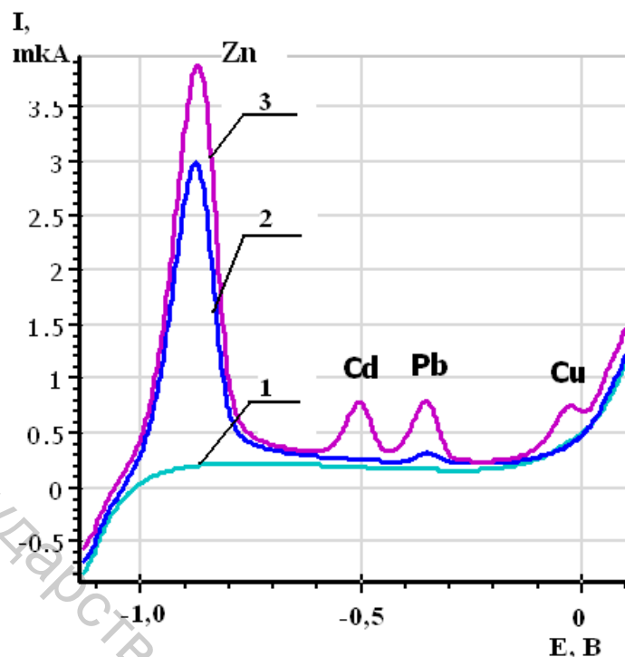
1 – фонового электролита ( 0,35 моль/дм 3 муравьиной кислоты); 2 – образца пробы сахара № 3; 3 – образца пробы сахара № 3 с добавкой стандартного раствора, содержащего по 2 мг/дм 3 Cd , Pb , Cu и 3 мг/дм 3 Zn . Температура раствора 25^{\circ}\text{C}
