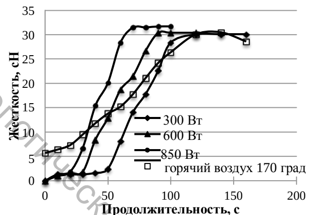
Рисунок 16 – Зависимость жесткости от продолжительности термофиксации
