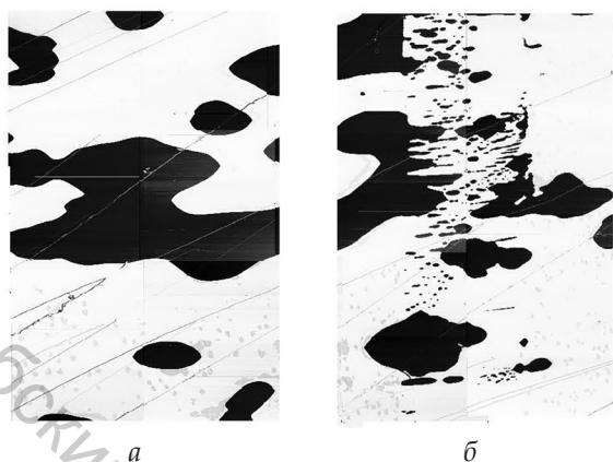
Рисунок 5 – Изображение доменной структуры (микроскопия пьезоотклика) кристаллов TGS-TGS+Cr , а – участок поверхности без примеси хрома, б – участок поверхности с полосой мелкодисперсной доменной структуры, соответствующей введению примеси хрома при выращивании кристалла. Площадь участков 78343,68 мкм 2
