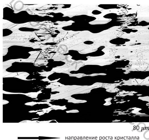
Рисунок 4 – Панорамное изображение доменной структуры кристаллов TFC-TFC+Cr , характеризующее изменение доменной структуры при нарастании кристалла от затравки к поверхности (слева направо). Пирамида роста {110}
