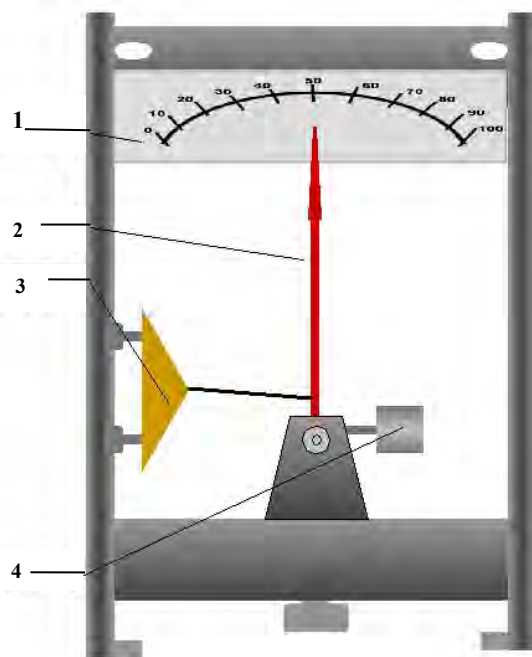
Рисунок 5.2 – Пленочный гигрометр: 1 – шкала; 2 – стрелка; 3 – мембрана; 4 – грузик
