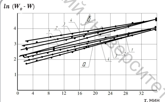
Рисунок 4 – Зависимости \ln(W_0 - W) = f(\tau) для сушки подошвенной кожи (а) и шерстяного войлока (б) при режимах, указанных на рисунках 1 и 2
