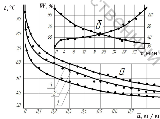
Рисунок 2 – Температурные кривые \bar{t} = f(\bar{u}) (а) и \bar{t} = f(\tau) и кривые сушки W = f(\tau) (б) для процесса сушки шерстяного войлока при режимах: 1 – t_c = 90 °C; v = 3 м / с; 2 – t_c = 120 °C; v = 5 м / с; 3 – t_c = 150 °C; v = 10 м / с
