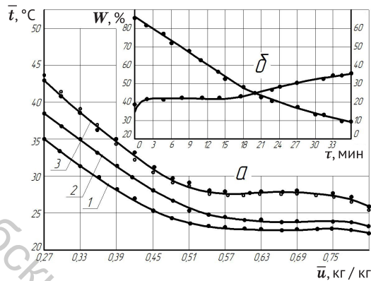
Рисунок 1 – Температурные кривые \bar{t} = f(\bar{u}) (а) и \bar{t} = f(\tau) и кривые сушки W = f(\tau) (б) для процесса сушки подошвенной кожи при режимах: 1 – t_c = 40 °C; v = 3 м / с; 2 – t_c = 50 °C; v = 5 м / с; 3 – t_c = 60 °C; v = 5 м / с
