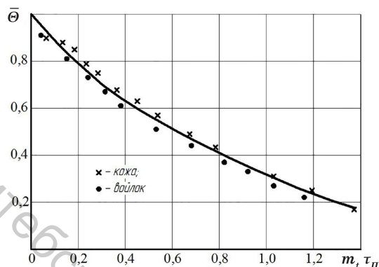
Рисунок 5 – Зависимость \bar{\Theta} = \exp(-m_t \tau_{\text{п}}) для сушки подошвенной кожи и шерстяного войлока при режимах, указанных на рисунках 1 и 2
