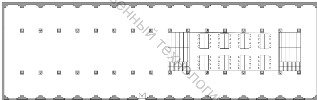
Рисунок Б.5 – План расстановки мебели и оборудования
