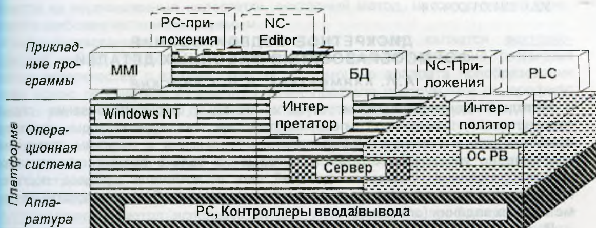
Рисунок 4 - Однокомпьютерный вариант системы PCNC
